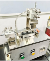
拉链片寿命测试仪
